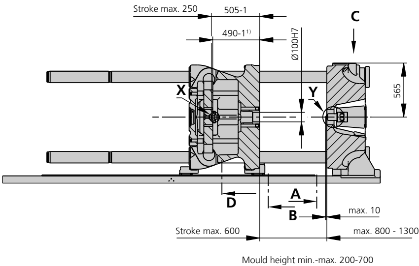
Ejector bolt | X
