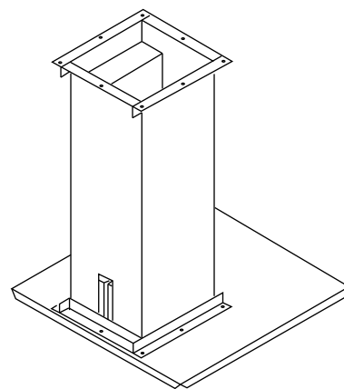
3 Attenuator
